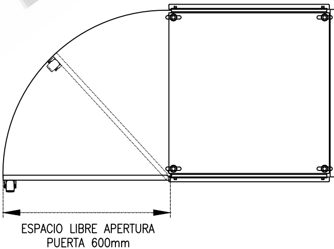
VISTA SUPERIOR APERTURA PUERTA A-A
