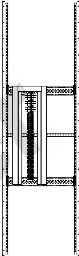
CORTE D-D' DETALLE DE BORNERA ①
