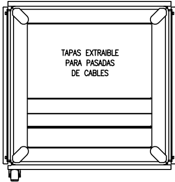
VISTA INFERIOR PASADA DE CABLES B-B
