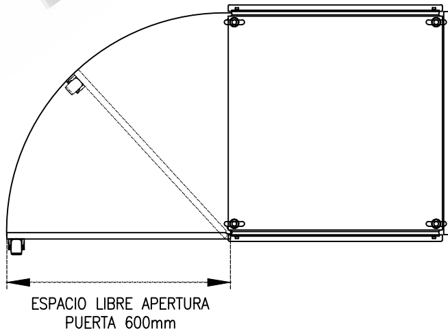
VISTA SUPERIOR APERTURA PUERTA A-A
